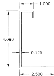
46 DAMPER JAMB 6063-T5 ALUMINUM
